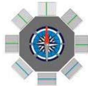
E-NE-N-NO-O : lames perpendiculaires au mur SO-S-SE : lames parallèles au mur
