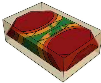
Effet de chaleur avec 2 côtés chauffés (surface de 6 x 4 m)
