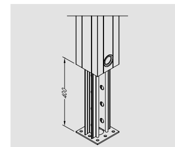
Pied de montage noyé
