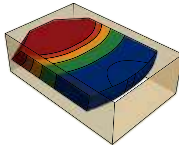
Effet de chaleur avec 1 côté chauffé (surface de 6 x 4 m)
