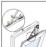
Kantelscharen inoliën
